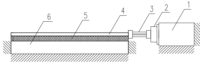
(b) 侧视图
