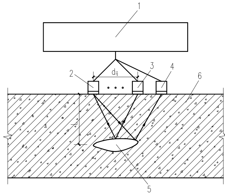
1—超声采集与分析装置；2—第 i 个超声发射换能器；3—第 j 个超声接收换能器； 4—第 j+1 个超声接收换能器；5—内部缺陷；6—钢筋混凝土； d_{ij} —第 i 个与第 j 个换能器的间距； L —缺陷深度
