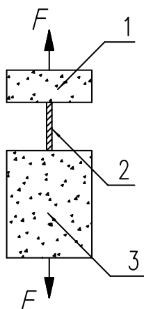
1—外叶板混凝土；2—保温拉结件；3—内叶板混凝土
