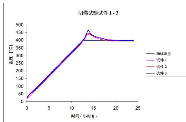
图 E.0.17-2 温度曲线示例
