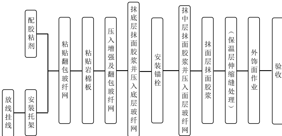
7.4.2 以锚为主岩棉板外墙外保温系统施工流程图
