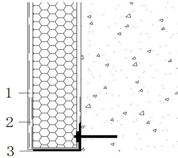
图 7.4.3 安装保温板起步托架
