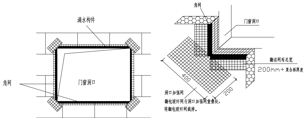
图 7.4.6 门窗洞口耐碱玻璃纤维网布加强图
