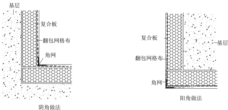
图 7.4.8 阴阳角角网设置示意图
