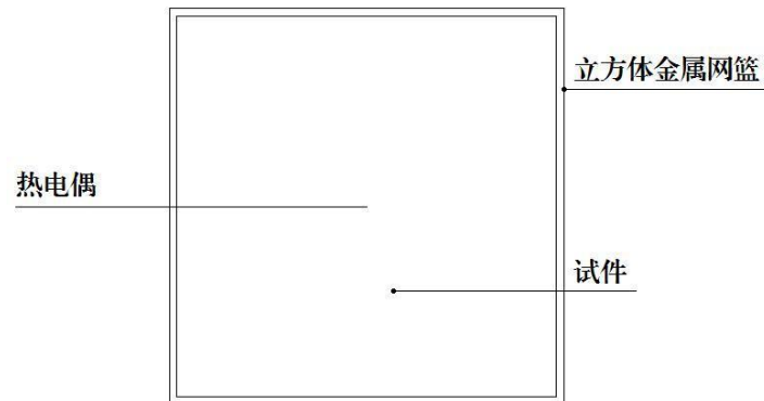
图 E.0.17-1 试件安装示意图
