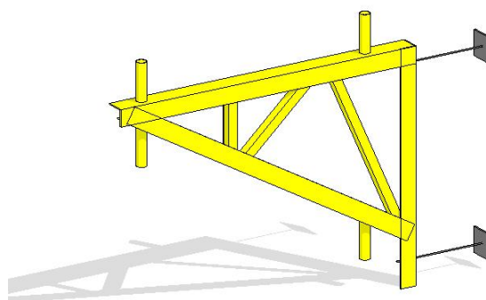
图 7.3.5-1 型钢悬挑架
